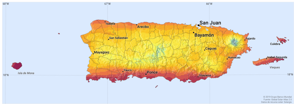
Promedios de largo plazo del potencial eléctrico fotovoltaico, periodo 1999-2018
